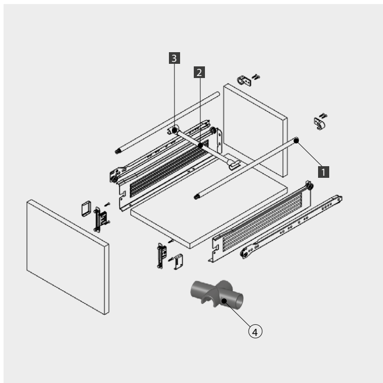
Релинг Smart Slide – Sam Box
