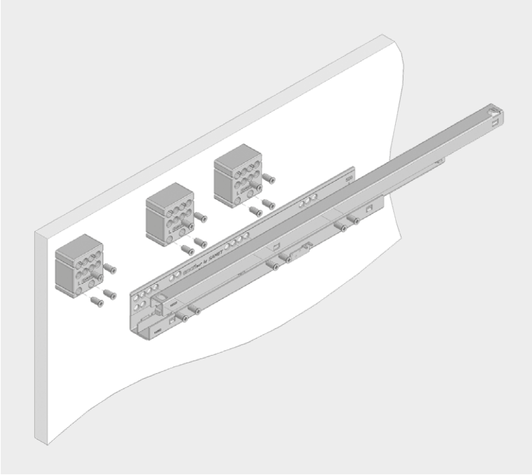
Расположение винтов для направляющих
