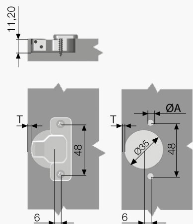
Тех.карта чашки 48 мм
