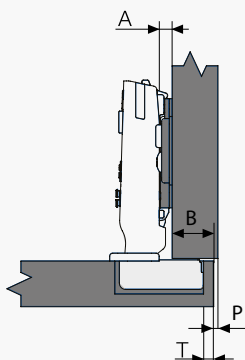
Накладная петля (0 мм)
