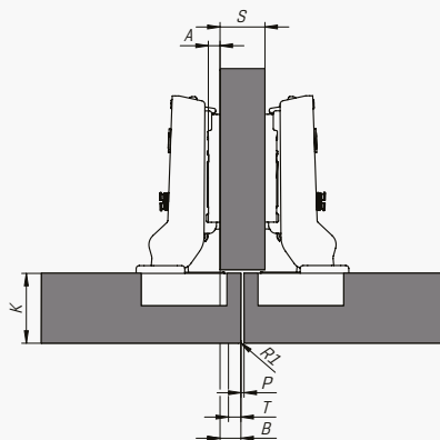
Полунакл. петля (9 мм)
