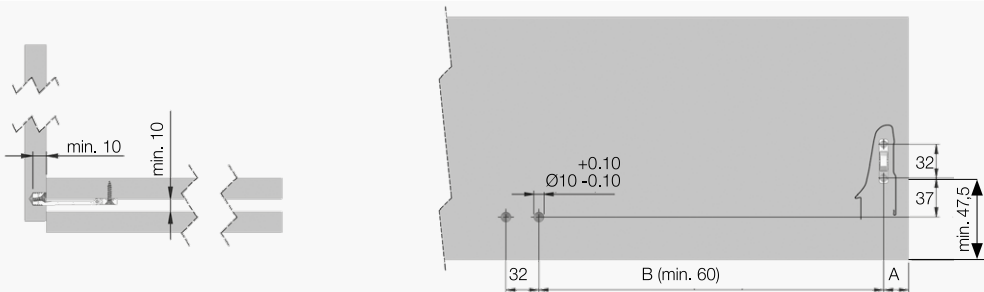
Размеры отверстий дна ящика
