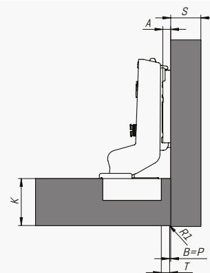
Вкладная петля (18 мм)
