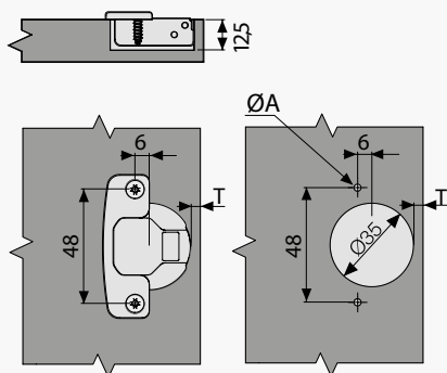
Тех.карта чашки 48 мм
