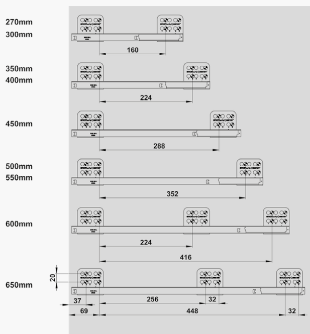
Разметка для направляющих
