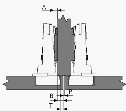
Полунакл. петля (9 мм)
