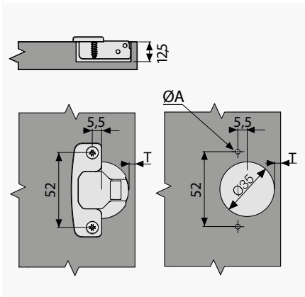
Тех.карта чашки 52 мм
