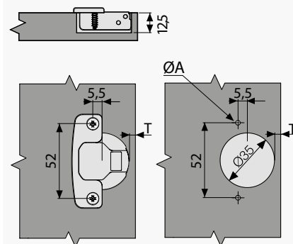
Тех.карта чашки 52 мм
