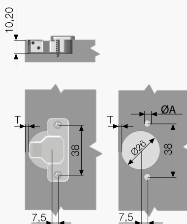
Тех.карта чашки 38 мм
