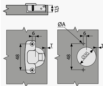
Тех.карта чашки 48 мм
