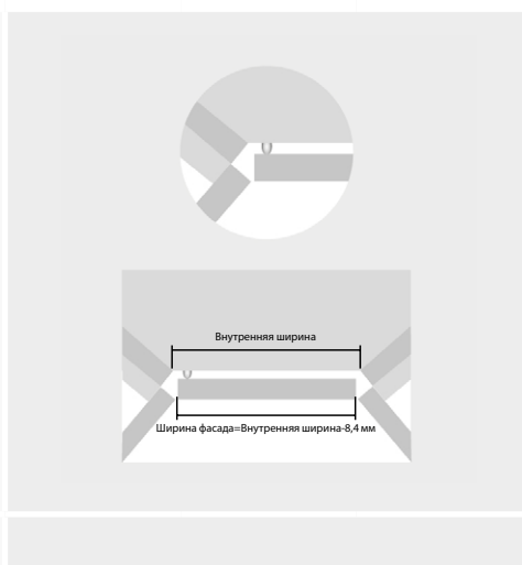
Тех.карта чашки 48 мм
