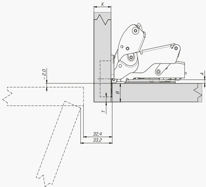
Накладная петля (0 мм)
