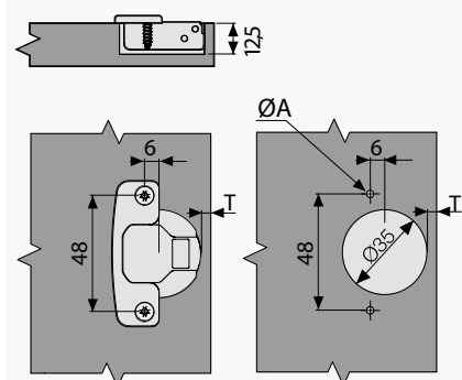
Тех.карта чашки 48 мм
