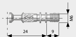
Дюбель M6x24 мм, сталь
