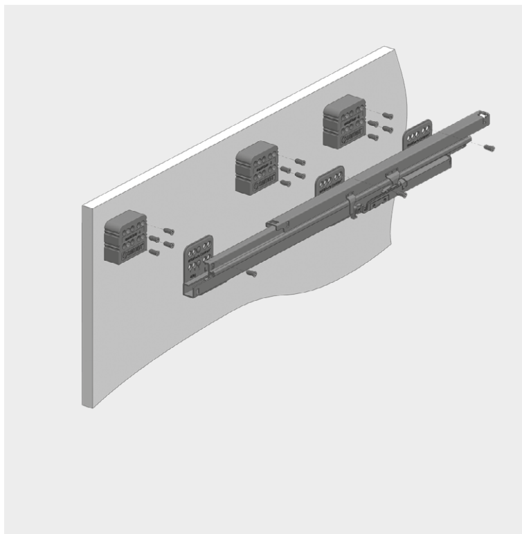
Разметка для направляющих
