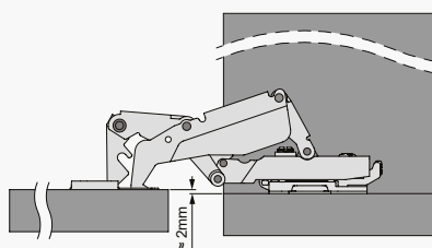
Установочные размеры
