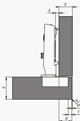
Накладная петля (0 мм)
