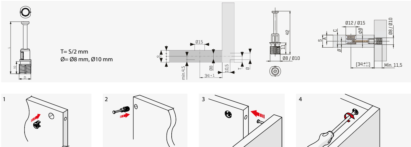
Установочные размеры
