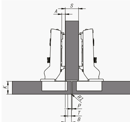
Полунакл. петля (9 мм)
