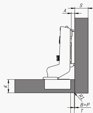
Вкладная петля (18 мм)
