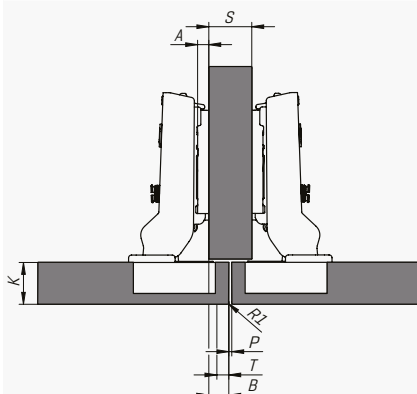
Полунакл. петля (9 мм)
