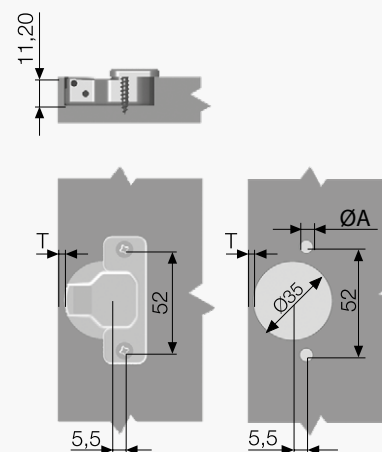
Тех.карта чашки 52 мм
