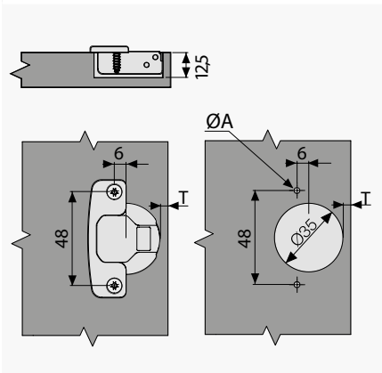
Тех.карта чашки 48 мм
