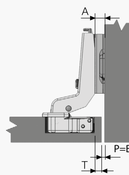
Вкладная петля (18 мм)
