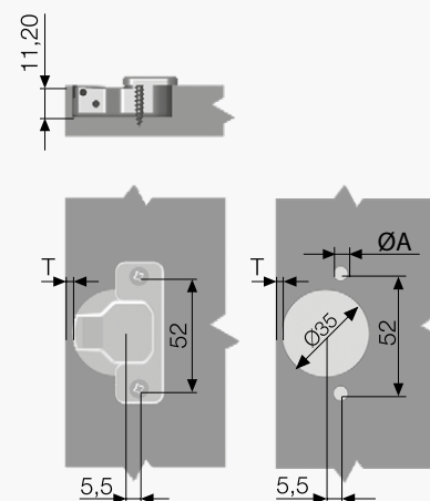
Тех.карта чашки 52 мм
