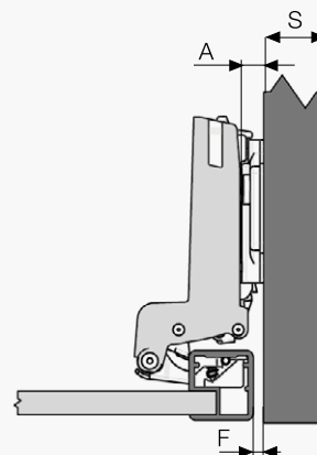
Вкладная петля (18 мм)
