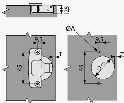
Тех.карта чашки 45 мм
