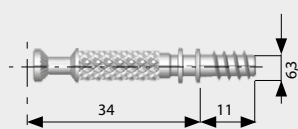
Дюбель 34 мм, сталь
