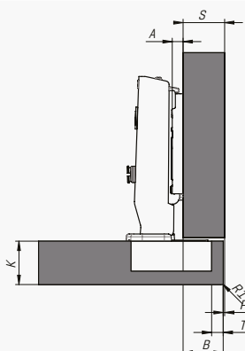
Накладная петля (0 мм)
