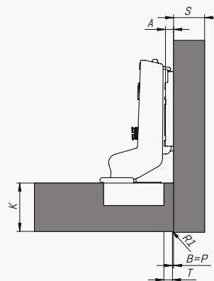
Вкладная петля (18 мм)
