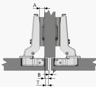
Полунакл. петля (9 мм)
