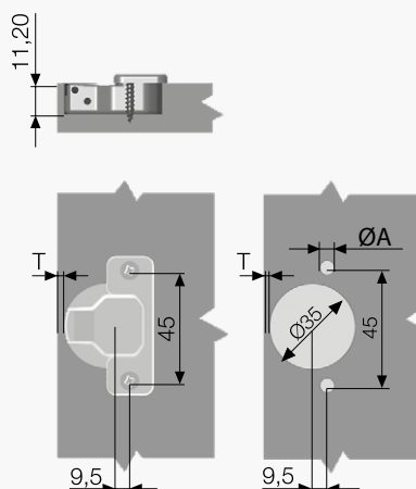
Тех.карта чашки 45 мм
