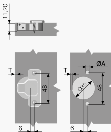
Тех.карта чашки 48 мм
