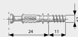
Дюбель 24 мм, сталь
