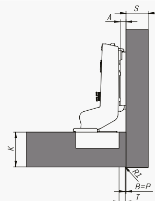
Вкладная петля (18 мм)
