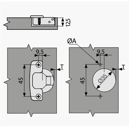
Тех.карта чашки 45 мм
