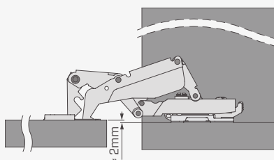
Установочные размеры
