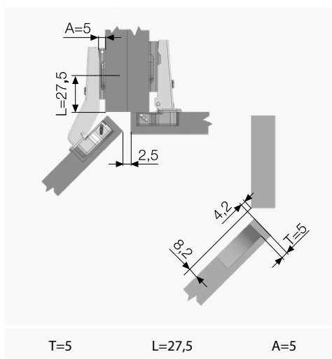
Тех.карта чашки 45 мм
