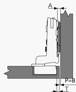
Вкладная петля (18 мм)
