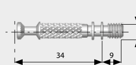
Дюбель M6x34 мм, сталь
