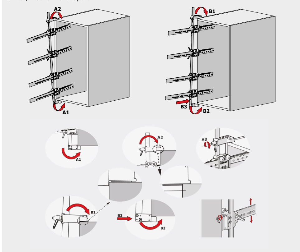
Фиксация с внешней стороны
