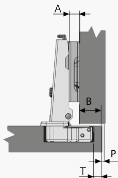
Накладная петля (0 мм)
