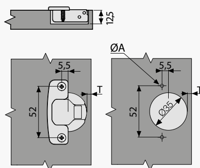
Тех.карта чашки 52 мм
