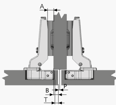
Полунакл. петля (9 мм)
