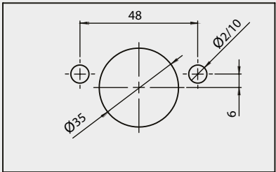
Сверлильные головки для петель
