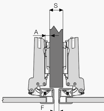
Полунакл. петля (9 мм)
