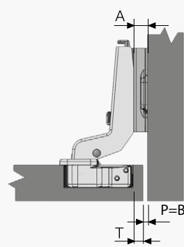
Вкладная петля (18 мм)
